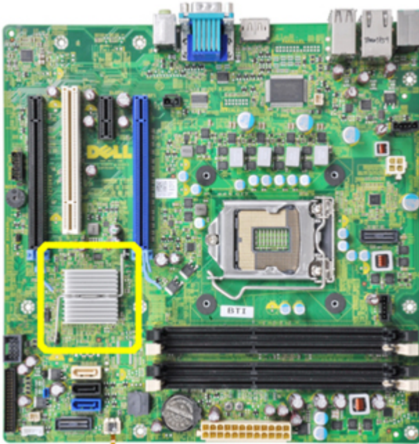
Ilustración 1. Placa base de una versión anterior con el disipador de calor.
