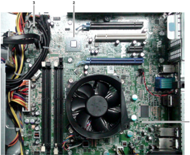
Ilustración 2. Placa base con el sensor térmico y el disipador de calor quitados
